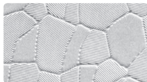
Austenit
